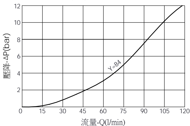
閥全開時雙向流量壓力曲線
