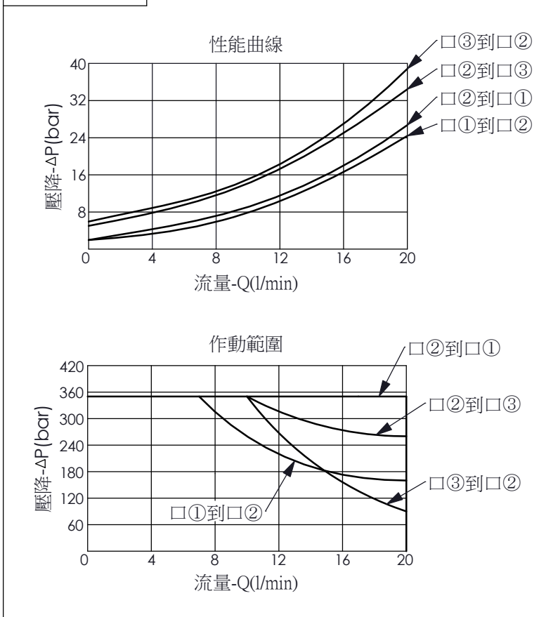
性能曲線圖
