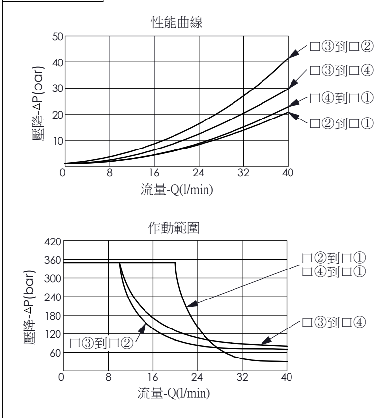
性能曲線圖
